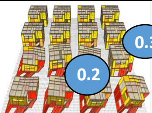
Wallstat地震倒壊シミュレーション
