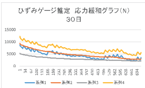
図 10 ひずみゲージ推定 応力緩和グラフ (N)
