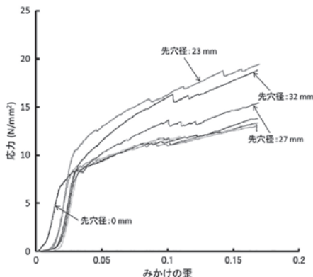
図 11 応力—みかけの歪曲線
