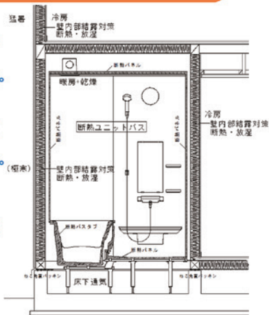
図6 断熱ユニットバス、「断熱・放湿」床下通気設計例
