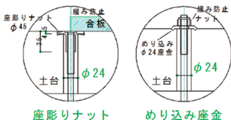
図 12 免震と減衰を発生させる、アンカーボルトの緊結法 (左: 根太レス床組み、右: 根太床組)
