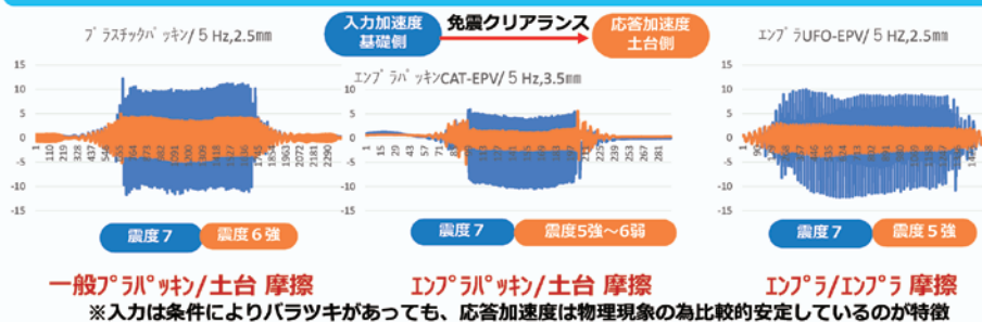
図8 時刻歴応答加速度グラフ / 「地震力>摩擦抵抗」の免震比較
