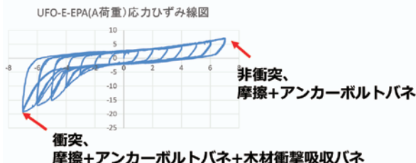
図9 土台下、地震力減衰グラフ
