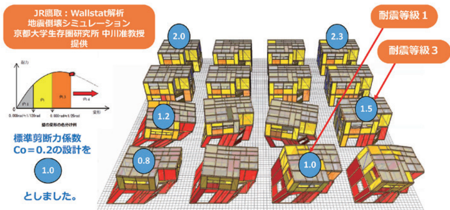
図2 耐震強度別地震倒壊シミュレーション
