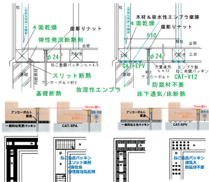
図5 在来プラスチック製ねこ土台とねこ土台型免震バッキンの比較図
