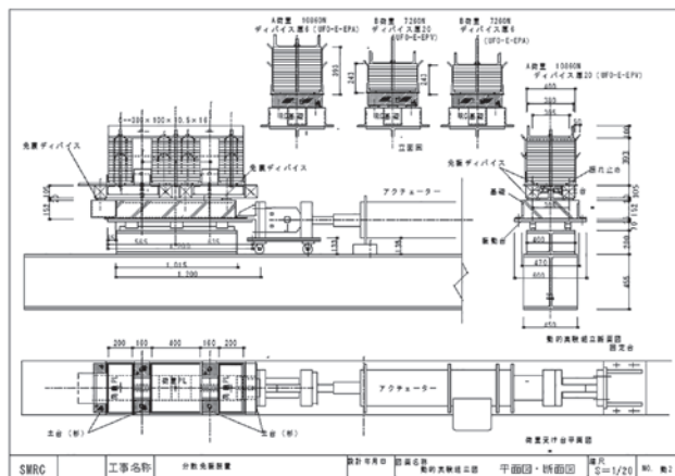
図7 RC基礎と木製土台の間に、摩擦アイソレータを挟んだ1質点系振動実験装置
